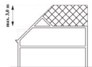
Doorsnede nokverhoging recht naar achteren uitgebouwd (op grotere kap)
