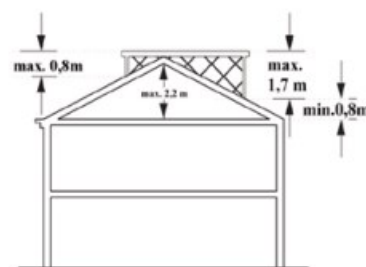
Doorsnede dakopbouw over de nok
