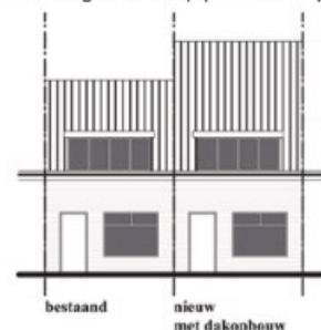
Aanzicht nokverhoging recht naar achteren uitgebouwd (op grotere kap)
