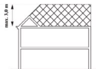
Doorsnede nokverhoging recht naar achteren uitgebouwd (op kleine kap)
