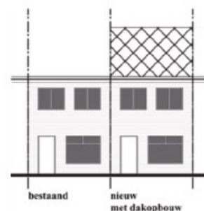
Aanzicht dakopbouw op plat dak
