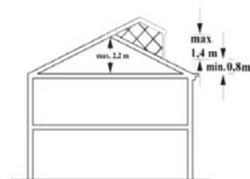
Doorsnede nokverhoging met kozijn bij een woning met symmetrisch zadeldak
