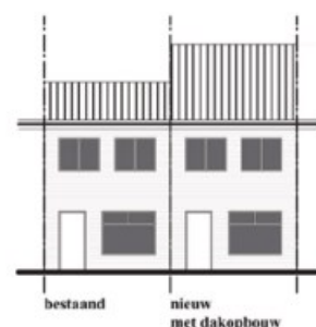
Aanzicht nokverhoging recht naar achteren uitgebouwd (op kleine kap)
