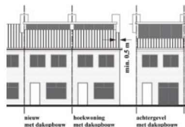
Aanzicht dakopbouw over de nok
